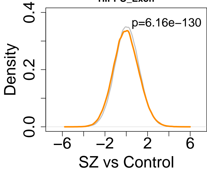
HIPPO_Exon
