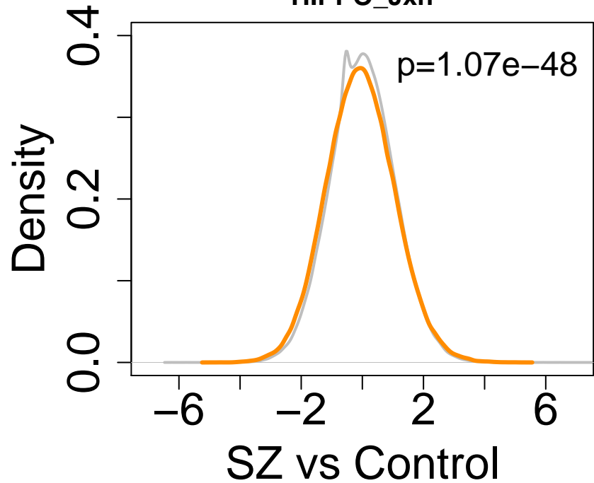
HIPPO_Jxn
