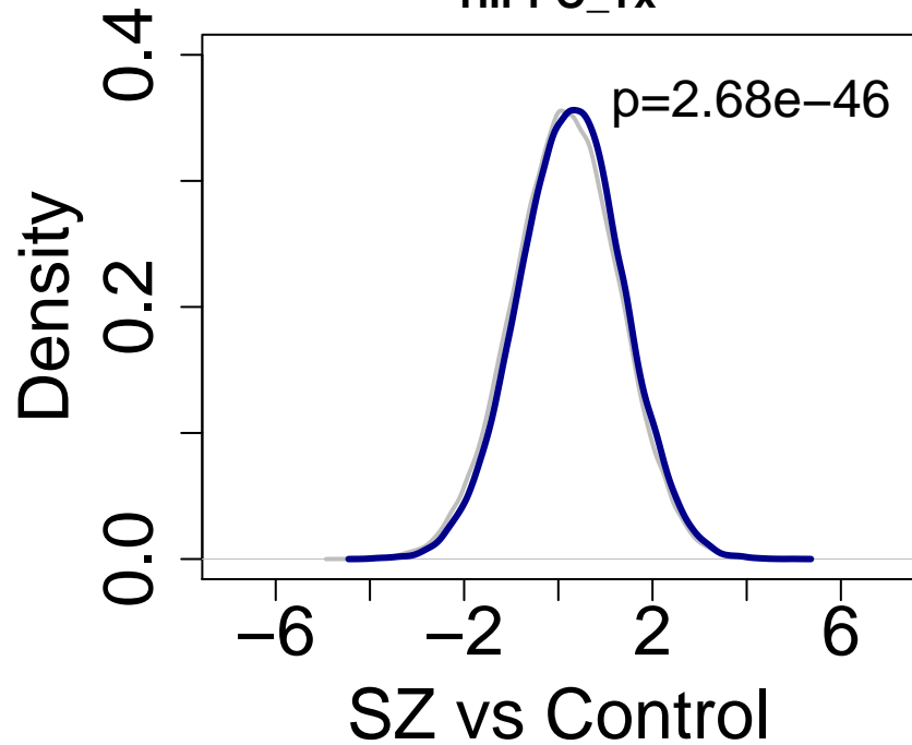
HIPPO_Tx
