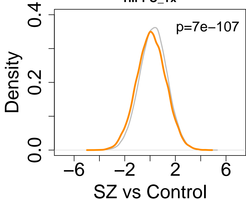
HIPPO_Tx
