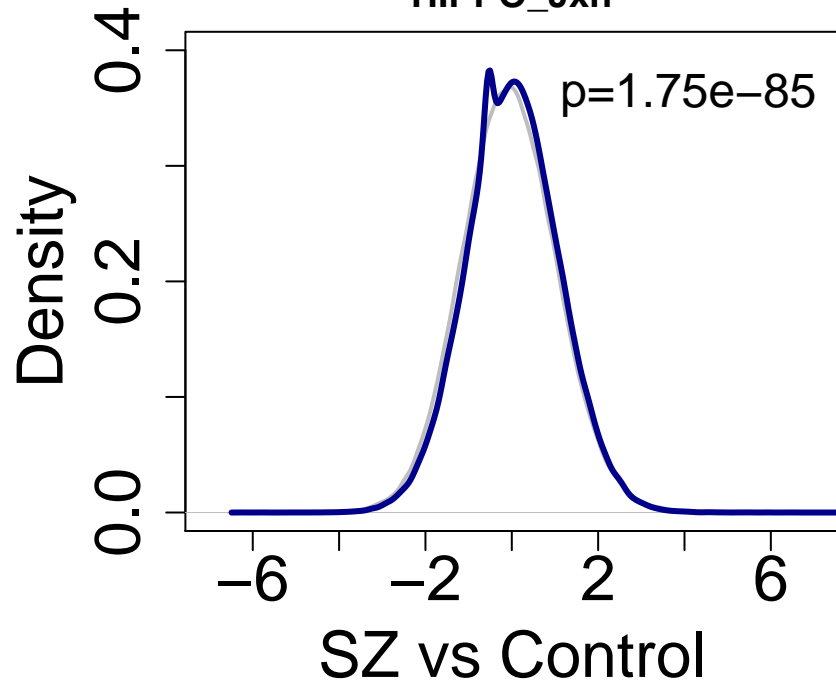
HIPPO_Jxn
