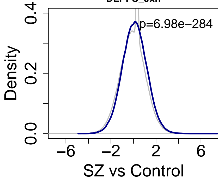
DLPFC_Jxn
