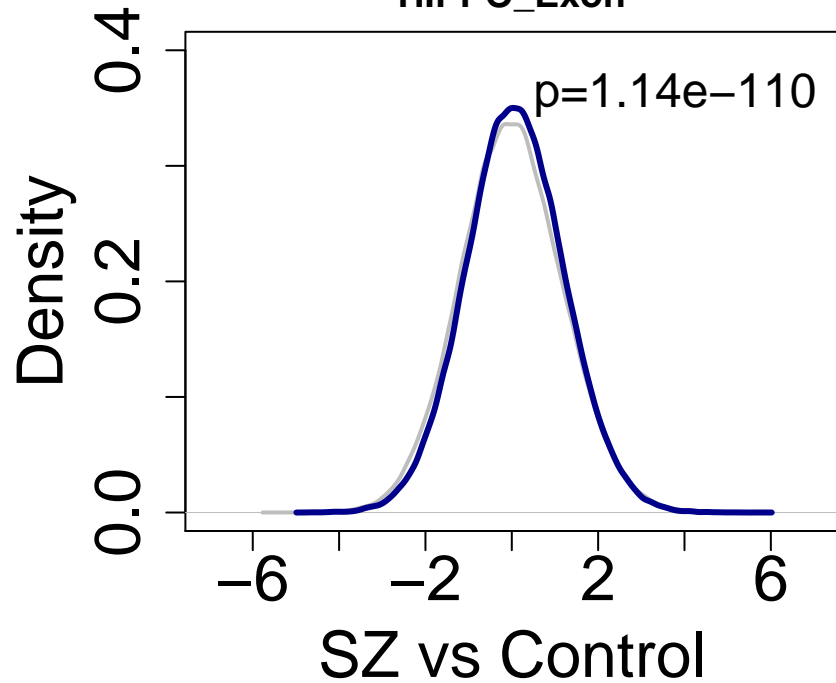
HIPPO_Exon
