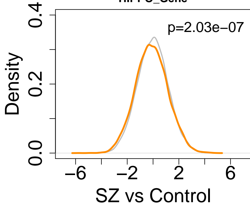
HIPPO_Gene
