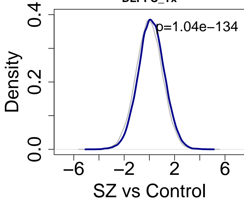
DLPFC_Tx
