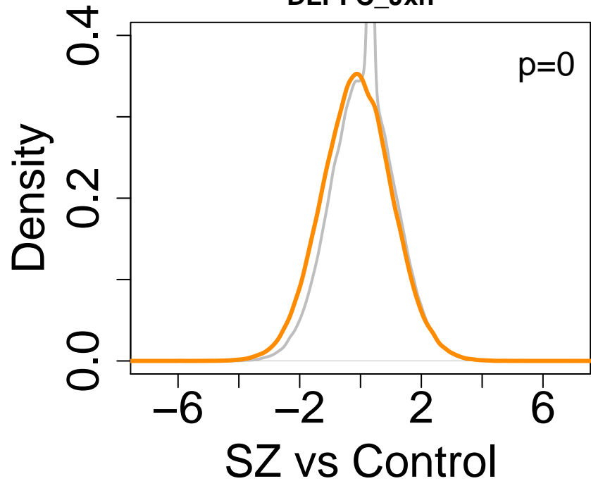
DLPFC_Jxn
